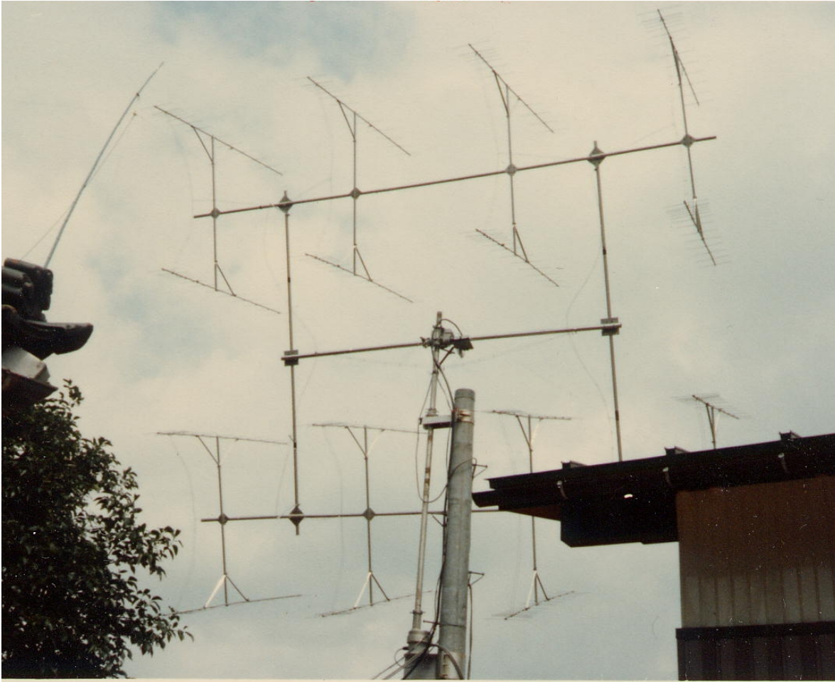
16 * K2RIW 13el Yagis 1980---1984
